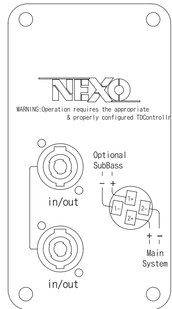
コネクターパネル拡大図
