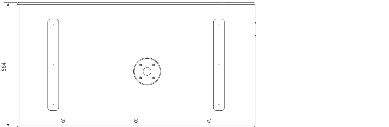
上面図
