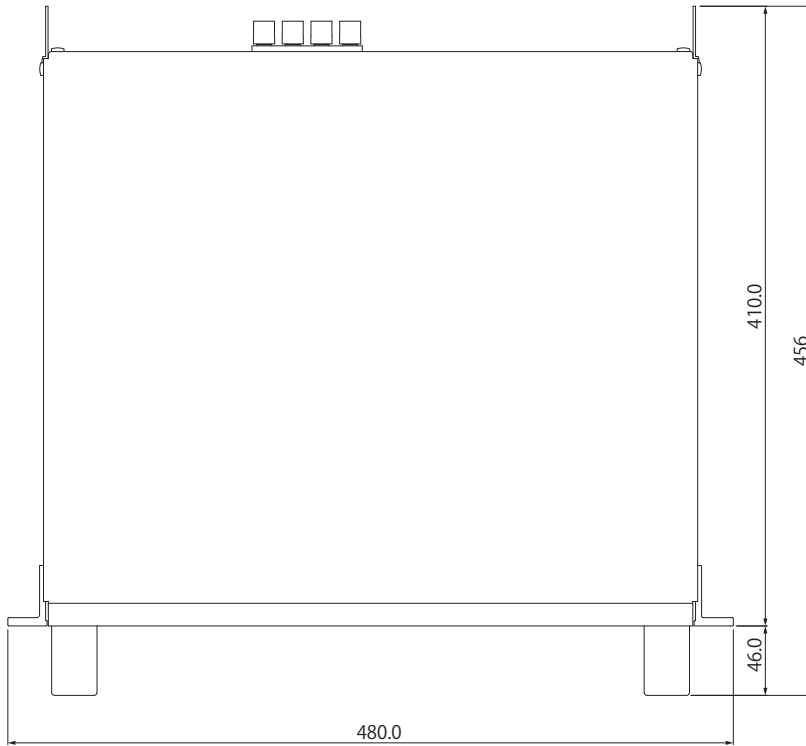
上面図
