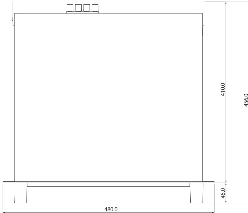
上面図
