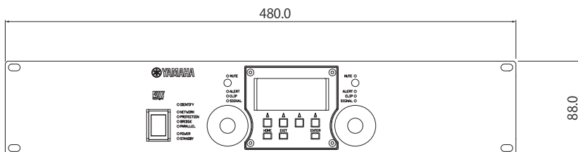
正面図
