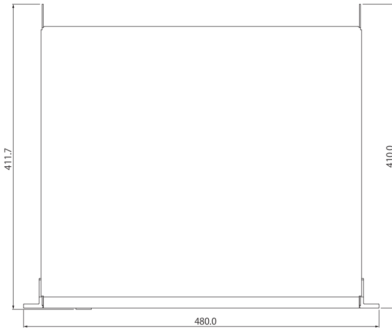
上面図
