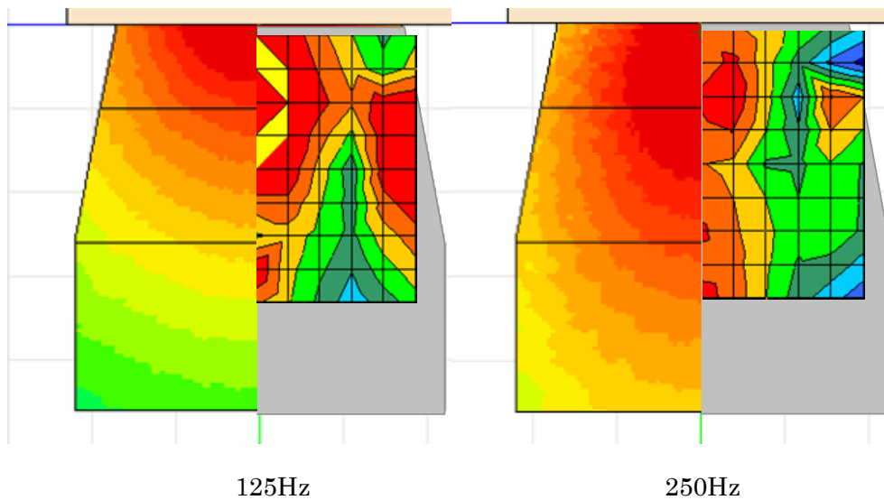
図 4: 周波数帯域ごとの音圧分布 (低音域) (左: Y-S 3 による計算結果、右: 実測結果)
